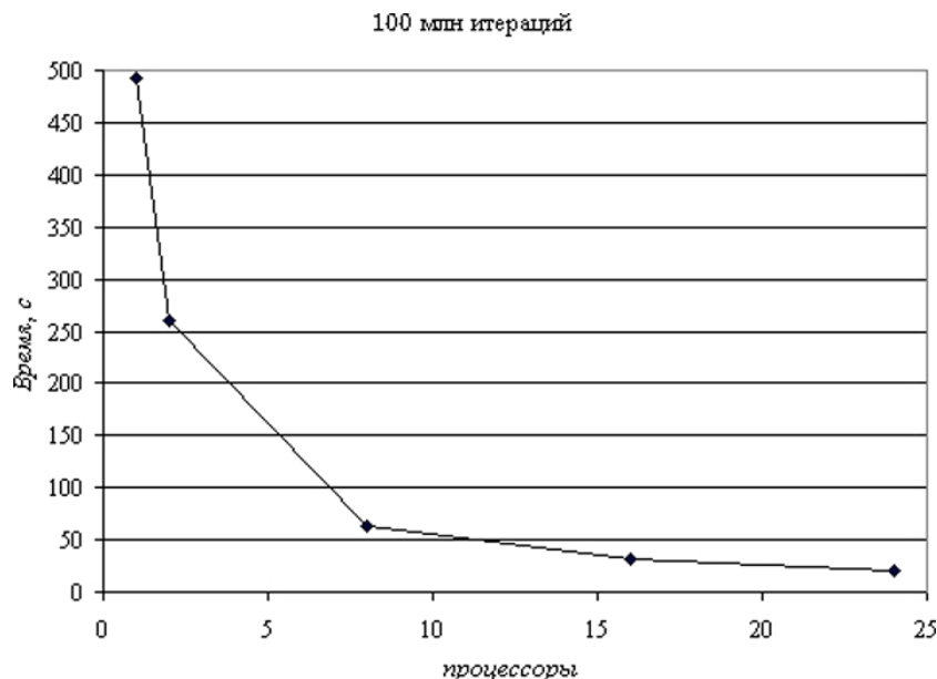
Рис. 1. Зависимость времени расчёта от числа процессоров
