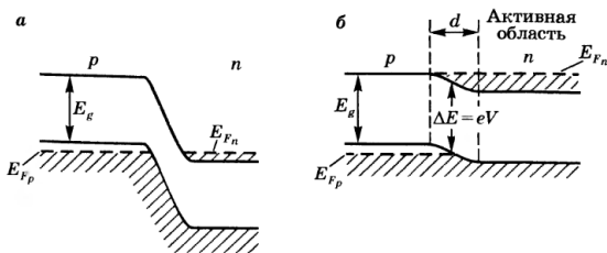
Рис. 3 Зонная диаграмма р-п перехода в отсутствие напряжения смещения (а), при прямом направлении (б)
