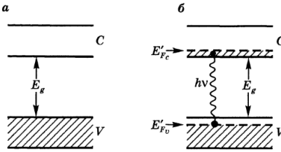
Рис. 2 Принцип работы полупроводникового лазера
