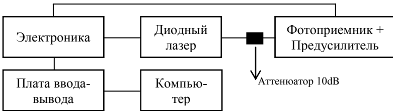
Рис. 11 Блок-схема установки
