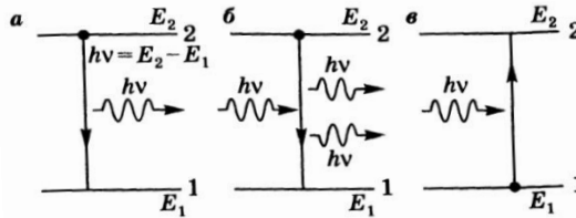
Рис. 1 Схематическая иллюстрация трех процессов: (а) спонтанного излучения, (б) вынужденного излучения, (в) поглощения
