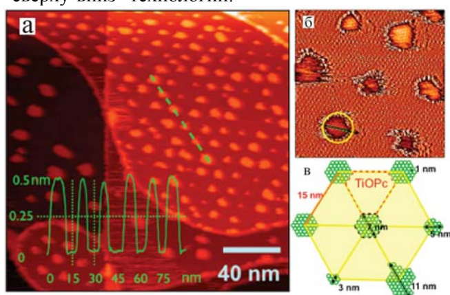
Рис. 2. а) СТМ-изображение фуллеренов C 60 , расположенных в вакансиях, образованных доменами TiOPc (на вставке изображена линия профиля шести фуллеренов C 60 , расположенных вдоль пунктирной линии); б) СТМ-изображение фуллеренов C 60 : отчетливо видны “ядро” из плотноупакованных фуллеренов и “кромка”, состоящая из менее связанных друг с другом кластеров C 60 ; в) схематическое изображение ансамблей фуллеренов C 60 и доменов TiOPc.
